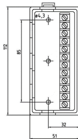
Unterteil mit Anschlussklemmen
